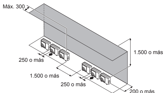
(1) Disposición de la unidad en un paralelo
