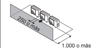
(2) Obstáculos en la parte delantera solamente
